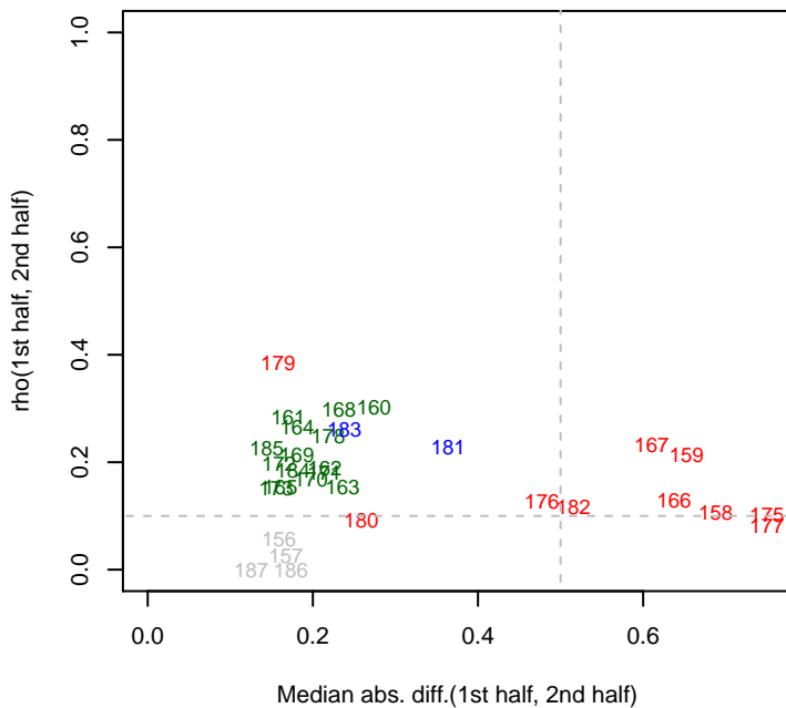
10/23/2013 Marino_ML2_set4 rho12
