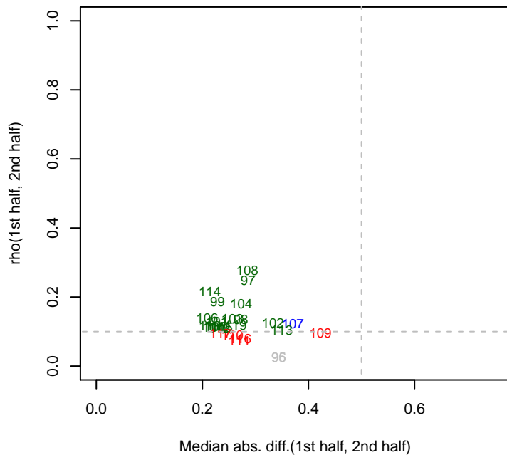
9/10/2013 Marino_ML2_set3 rho12
