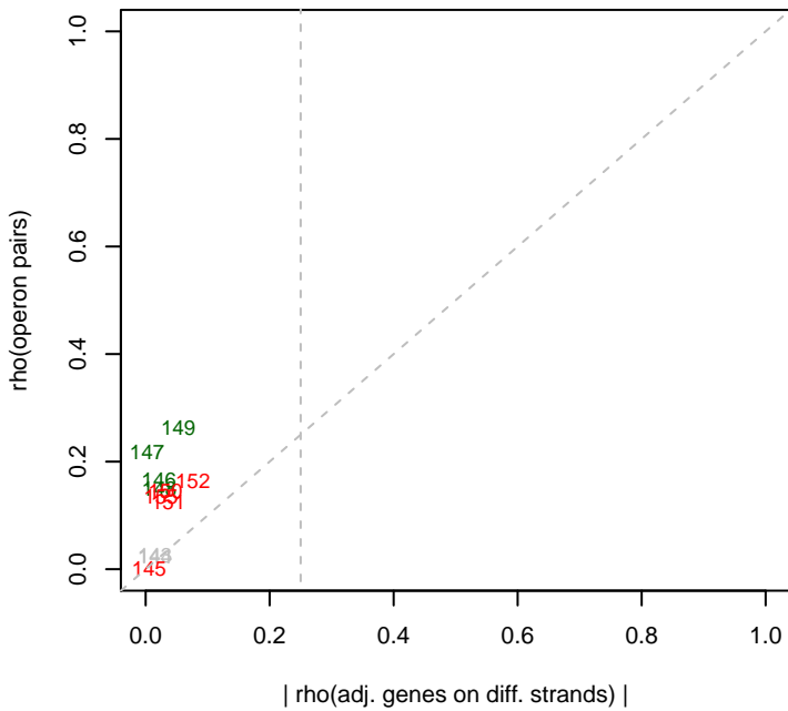
9/12/2013 Marino_Dino_extra_set rho(operons)
