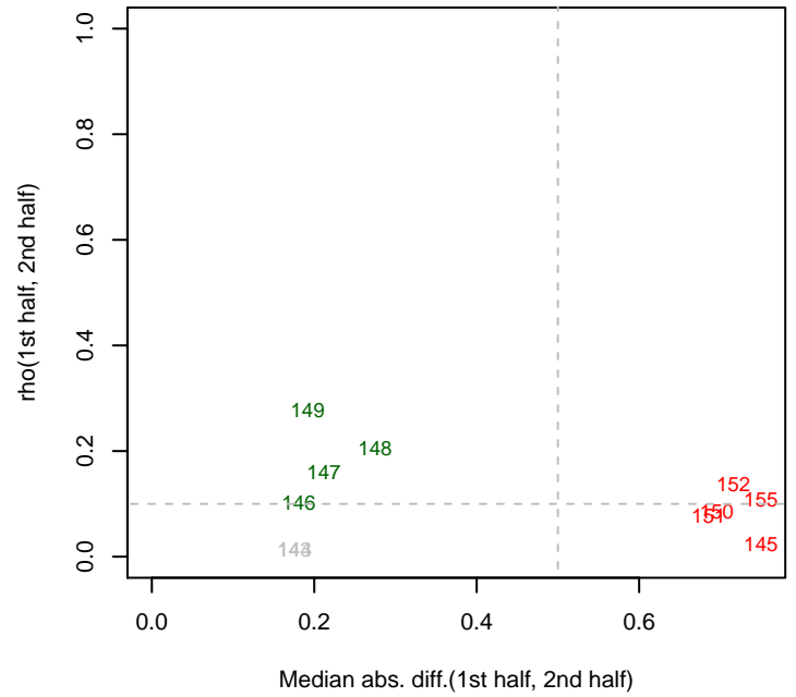
9/12/2013 Marino_Dino_extra_set rho12
