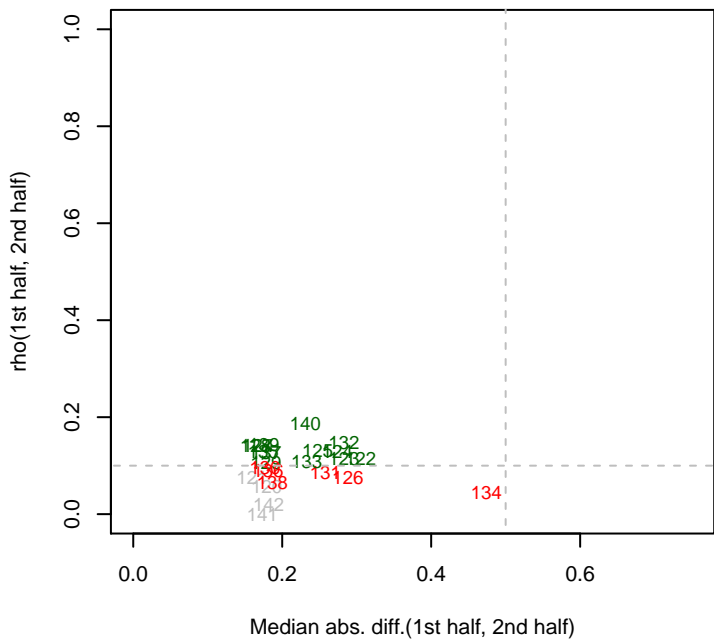
9/11/2013 Marino_ML2_set3 rho12
