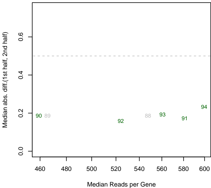
9/10/2013 Marino_ML2_set2 mad12
