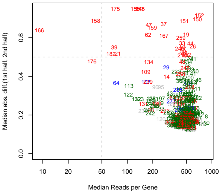
Marino mad12
