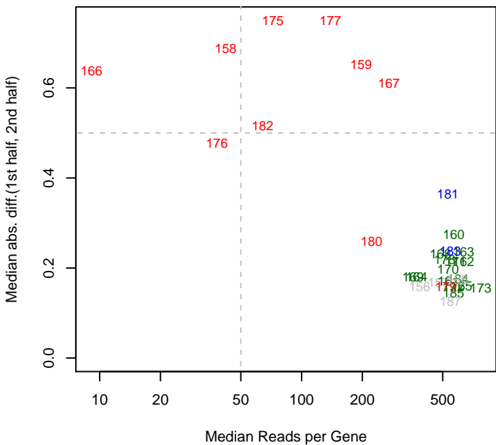
10/23/2013 Marino_ML2_set4 mad12
