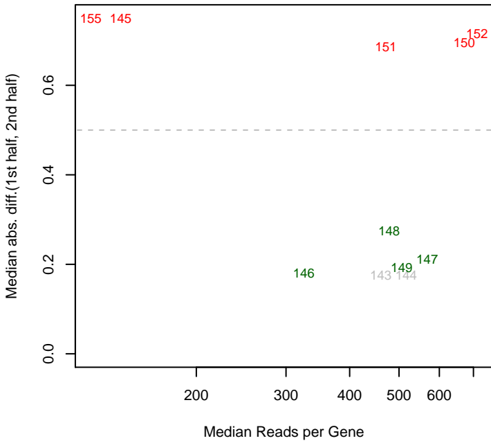
9/12/2013 Marino_Dino_extra_set mad12
