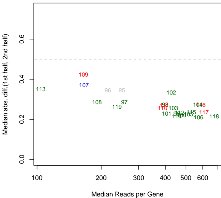
9/10/2013 Marino_ML2_set3 mad12
