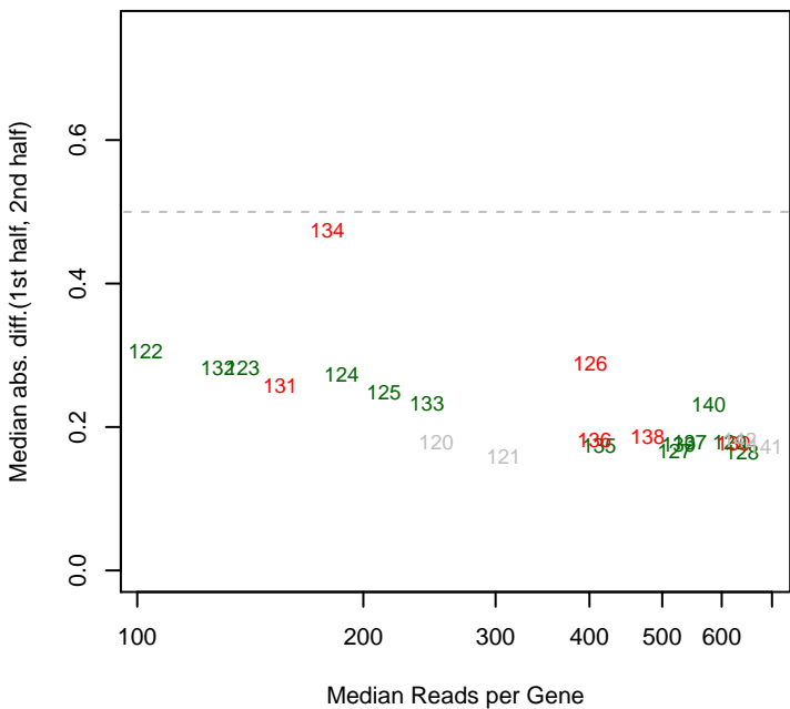
9/11/2013 Marino_ML2_set3 mad12
