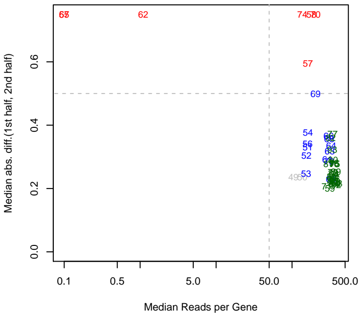
12/11/2013 PV4_ML1_set2 mad12
