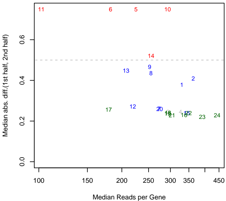
12/11/2013 PV4_ML1_set1 mad12
