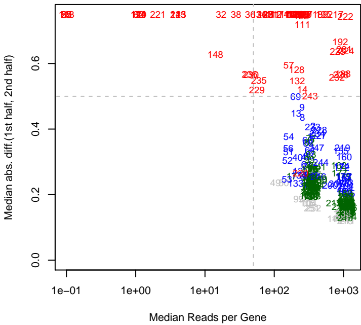
PV4 mad12
